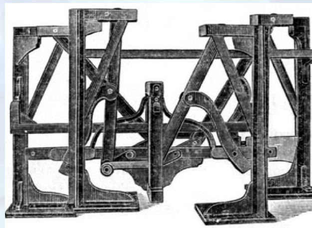
Стопоходящая машина
