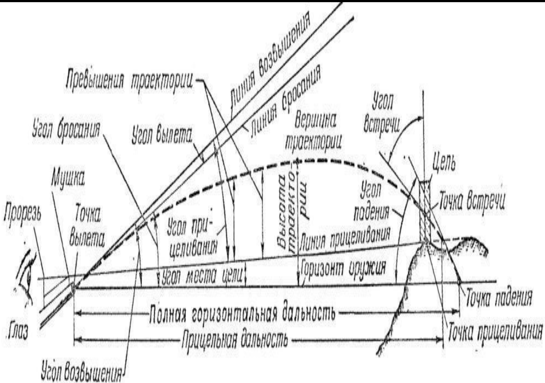
Рис.9 . Элементы траектории
