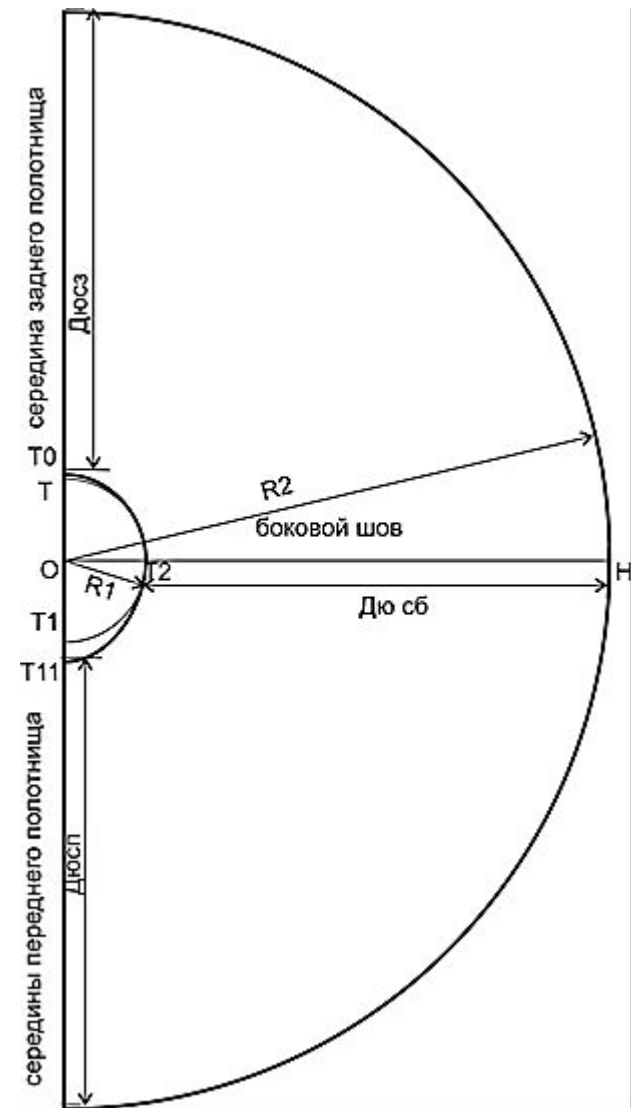
Чертеж конструкции юбки «полусолнце»
