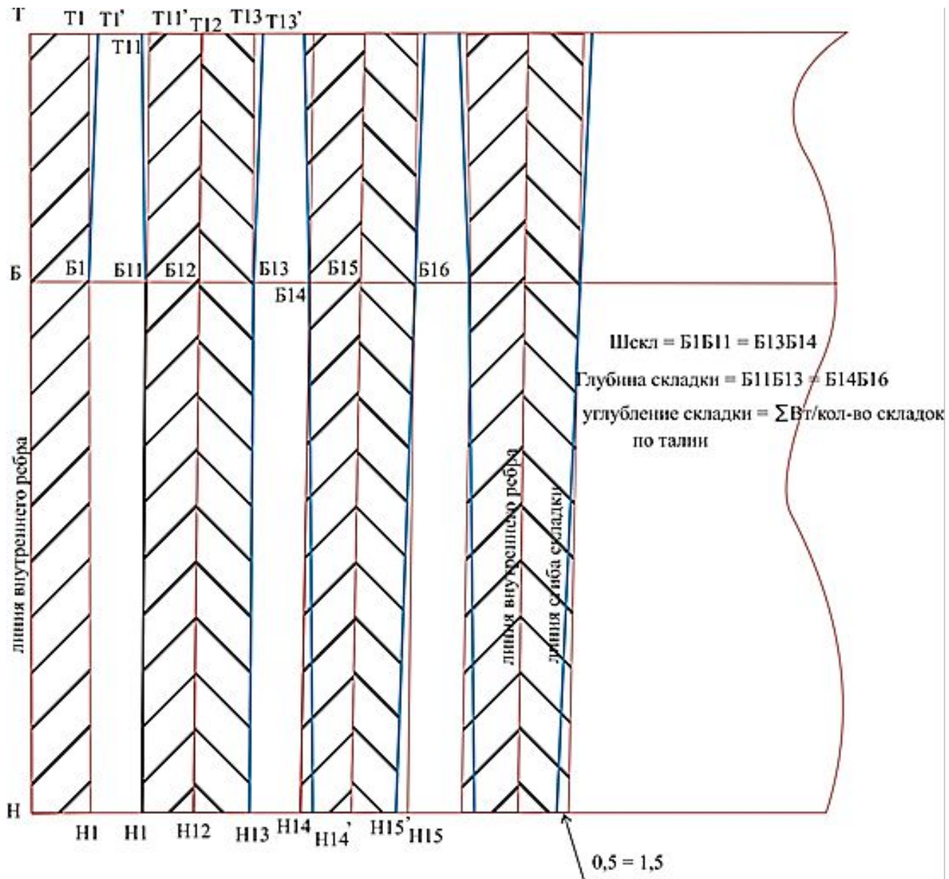
Чертеж построения юбки в круговую складку
