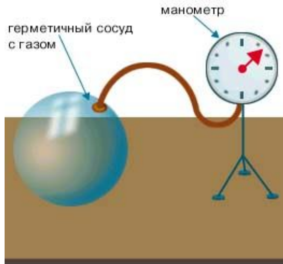
Газовый термометр.
