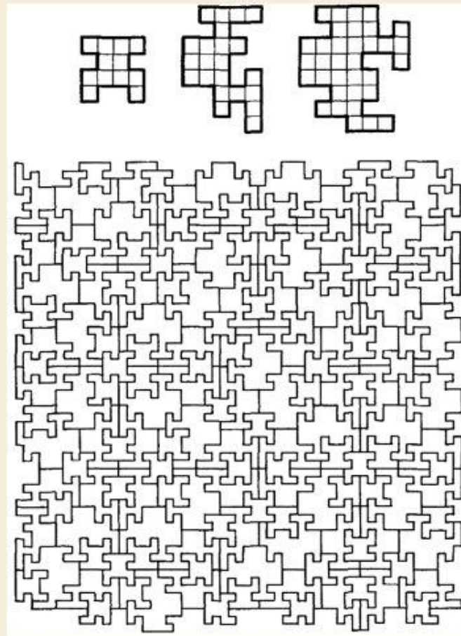
Рис. 1.3. Набор из трех полиоминo, покрывающий плоскость аperiodически (получен из
