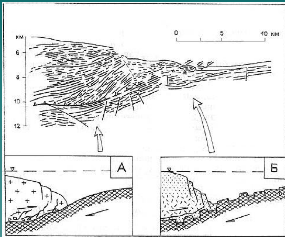
Механизмы тектонической эрозии: базальный (А), фронтальный (Б)
