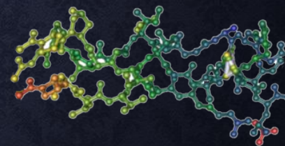
молекула ГИДРОЛИЗАТА КОЛЛАГЕНА
