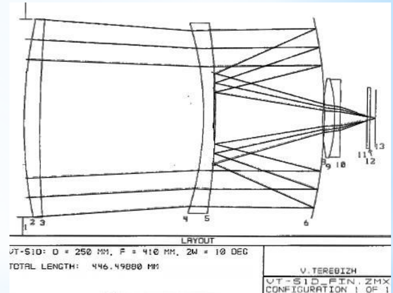
Объектив Сова 25
