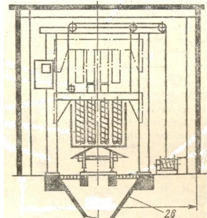
Бурорыхлительная установка
