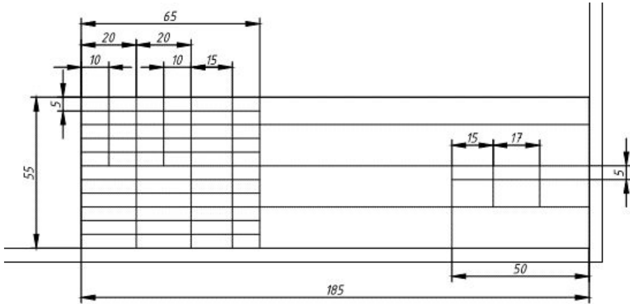
Основная надпись для строит.чертежей.
