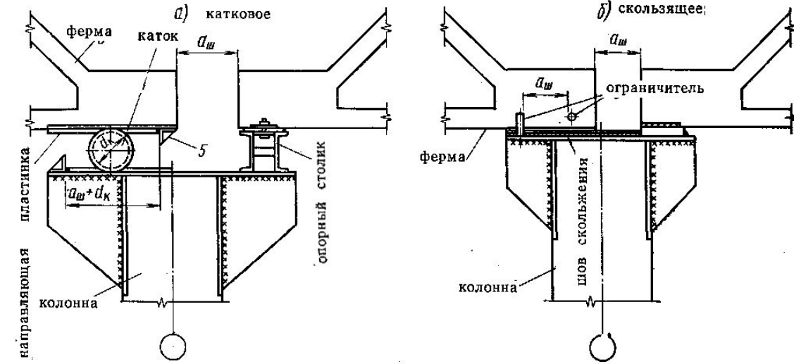
Шарнирно-подвижные сопряжения несущих конструкций покрытий с колоннами.
