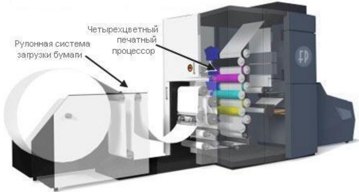
Цифровая печатная машина с рулонной загрузкой бумаги и возможностью двухсторонней печати
