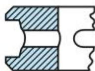
Маслосъемное кольцо коробчатого типа без пружинного расширителя
