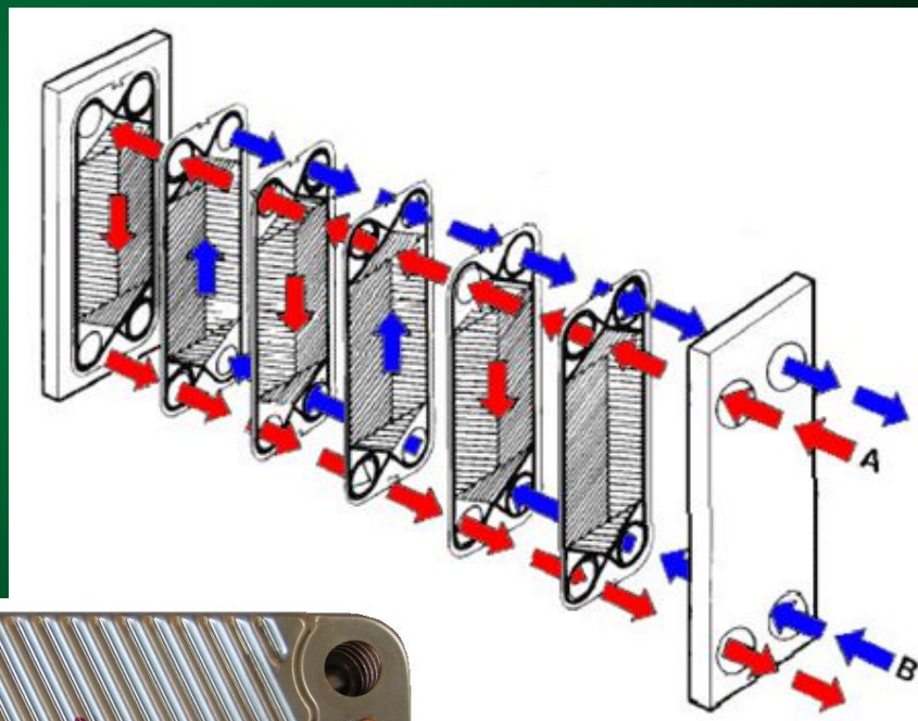
Пластины теплообменника
