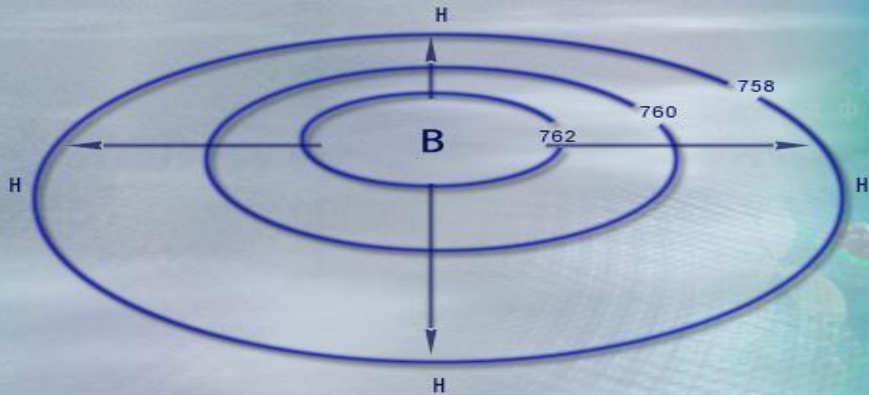
АНТИЦИКЛОН
