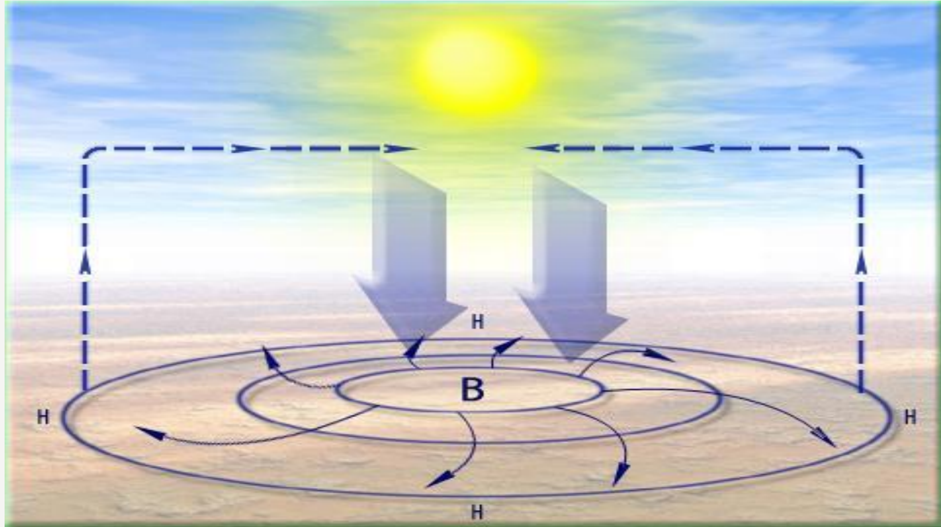
АНТИЦИКЛОН
