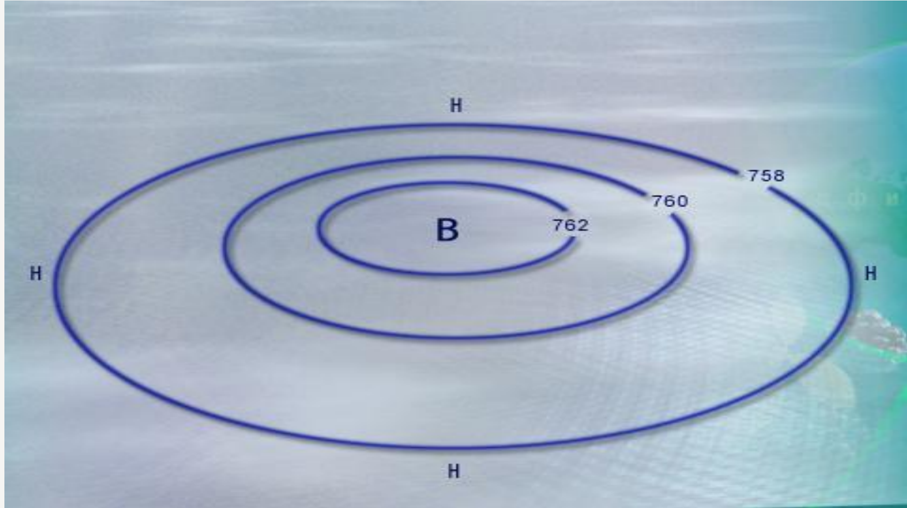
АНТИЦИКЛОН
