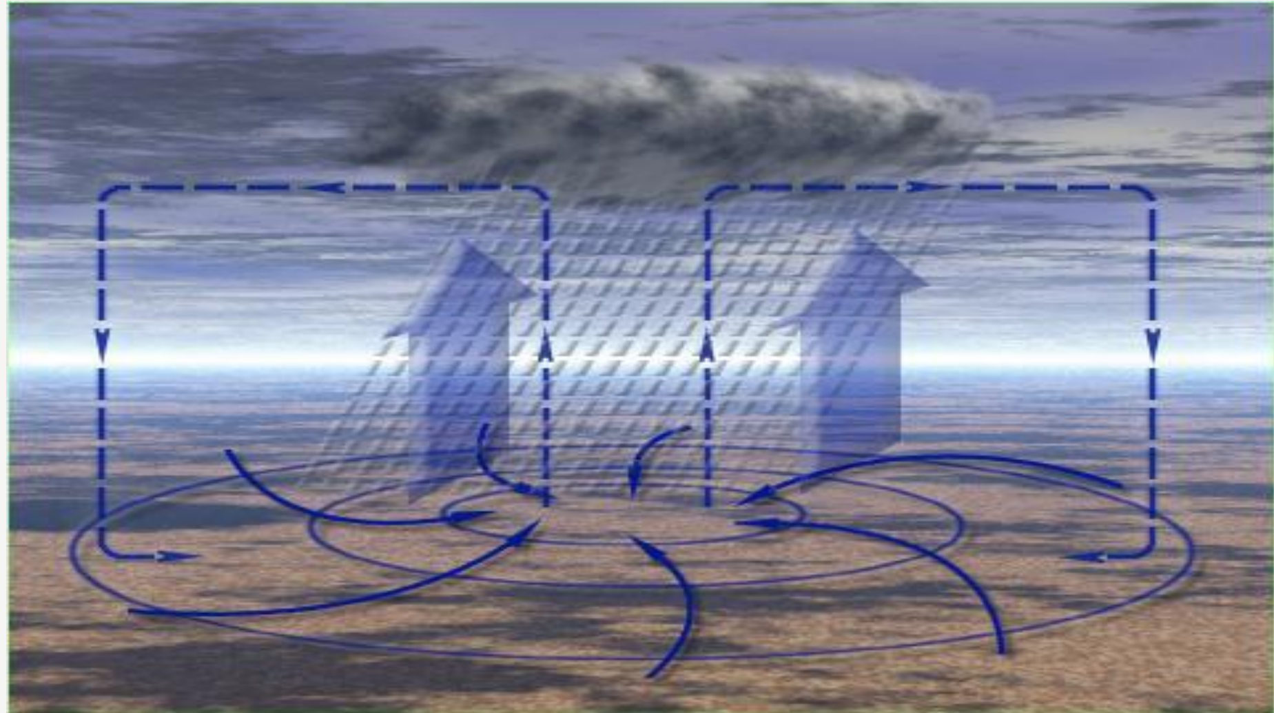
ЦИКЛОН
