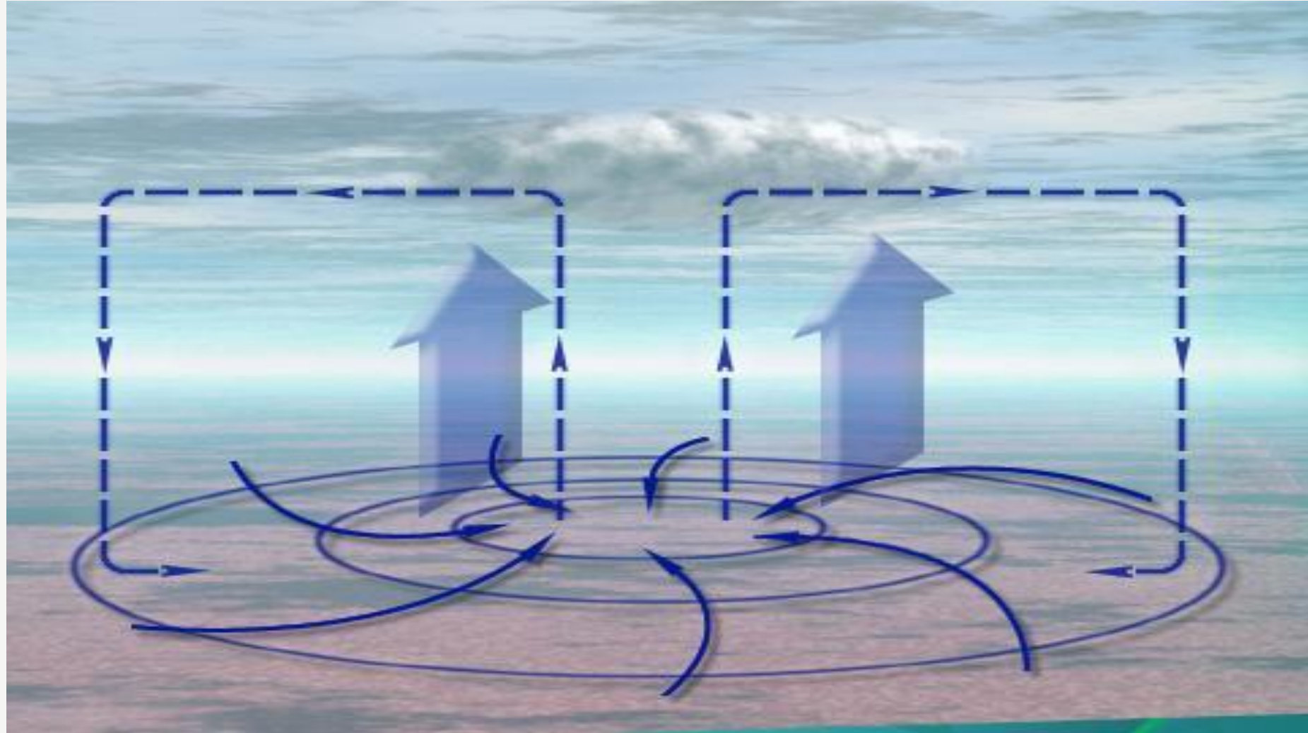
ЦИКЛОН
