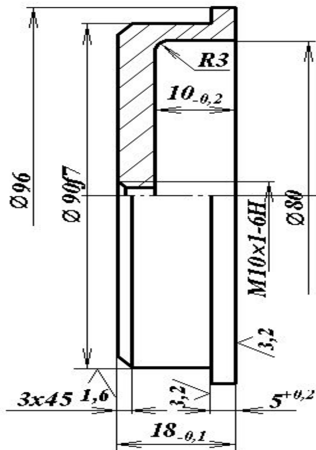
Рисунок 1.1 – Эскиз крышки.
