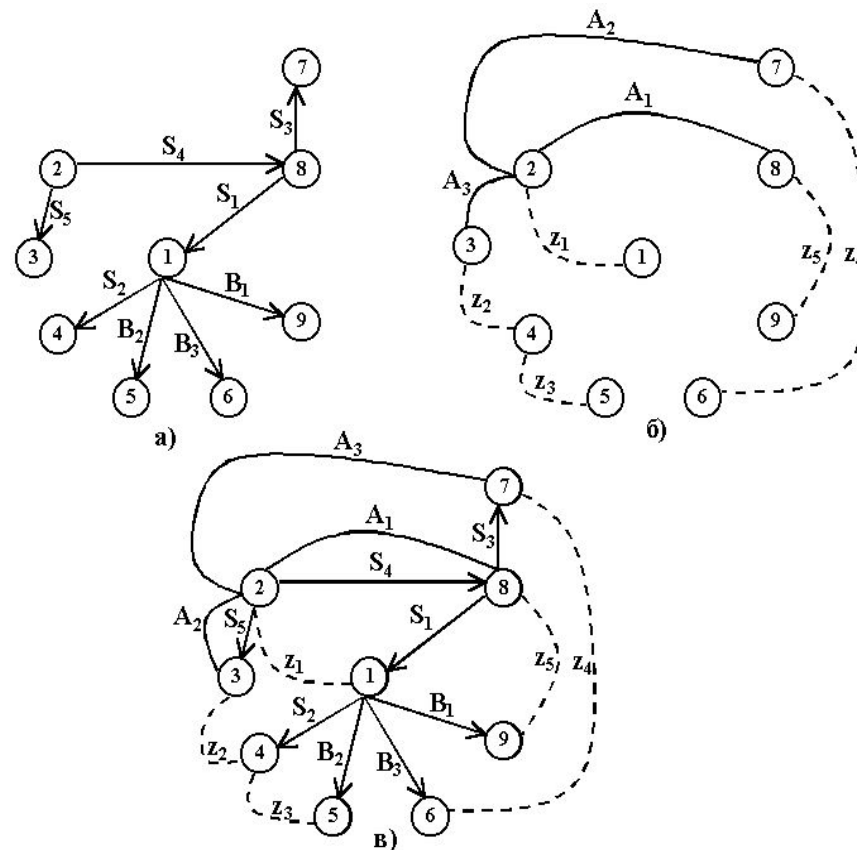
Рисунок 3.2 – Граф размерных связей технологического процесса. а) производное дерево, б) исходное дерево, в) совмещенный граф.
