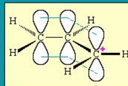
\text{CH}_2 = \text{CH} - \text{CH}_2^+ аллил-катион
