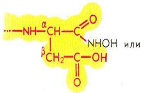
\alpha -Аспартилгидроксамаг
