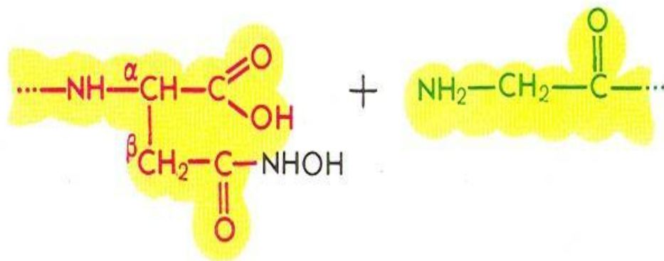
\beta -Аспартилгидроксамаг
