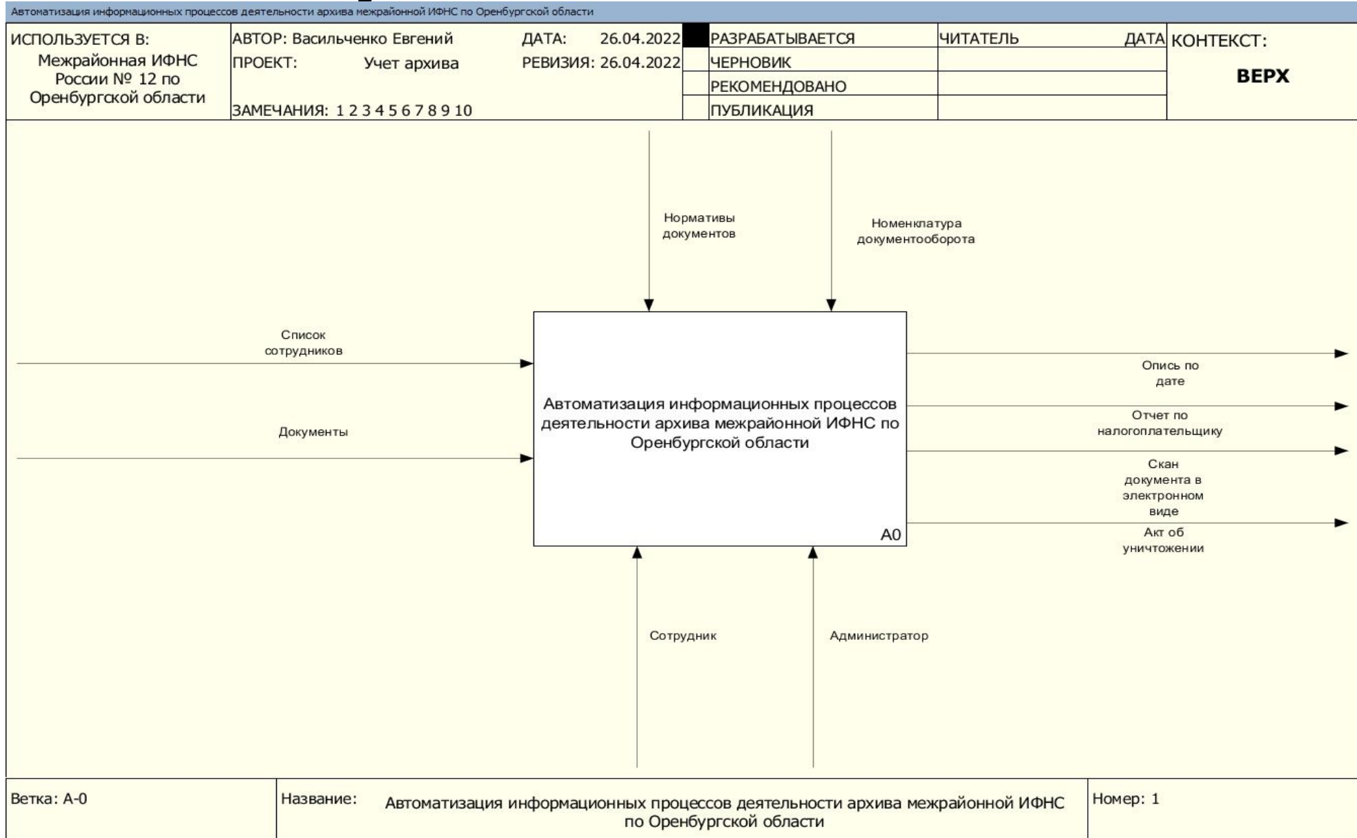
Рисунок 1 - Контекстная диаграмма
