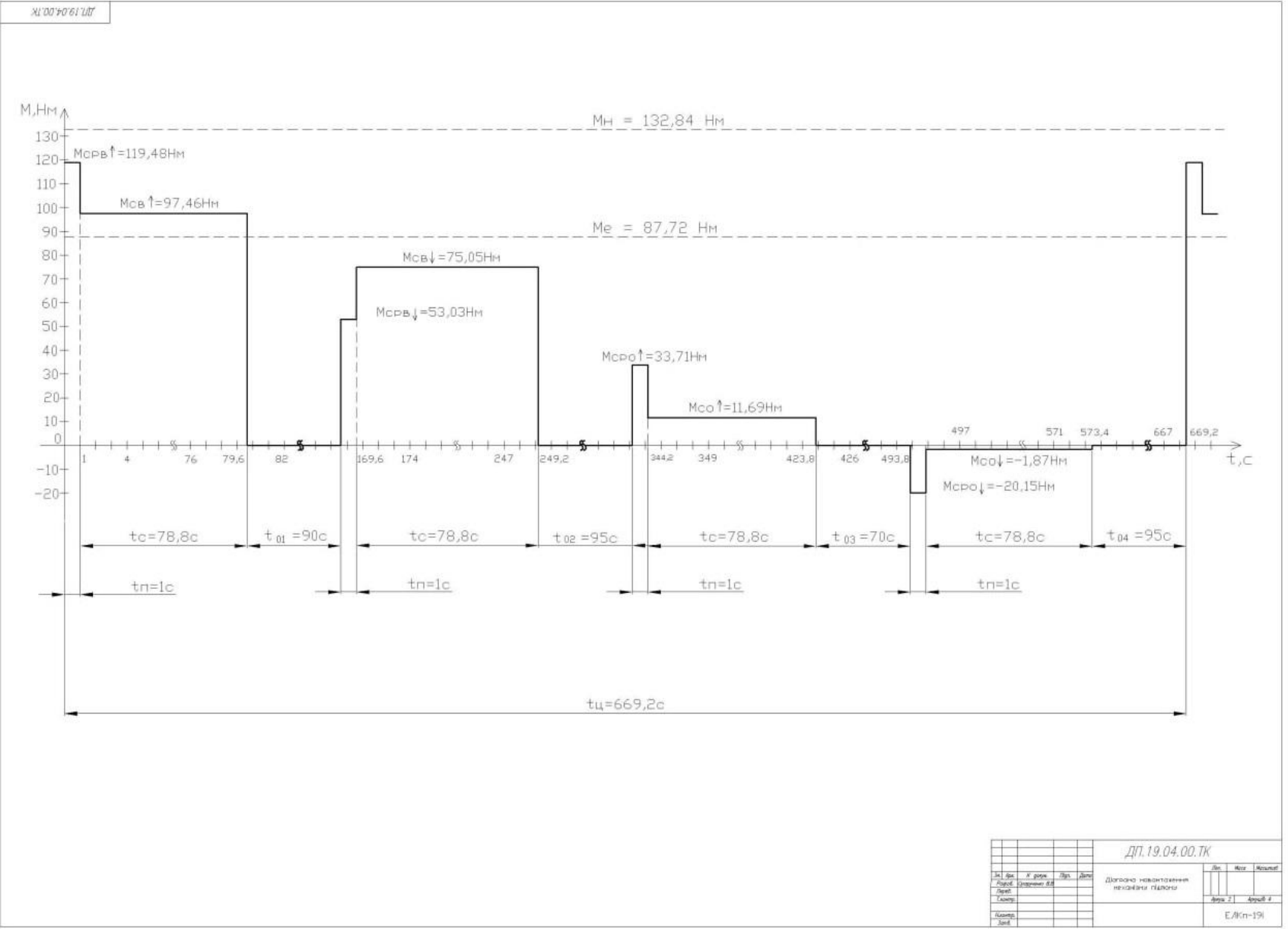
Рисунок 2 – Діаграма навантаження механізму підйому
