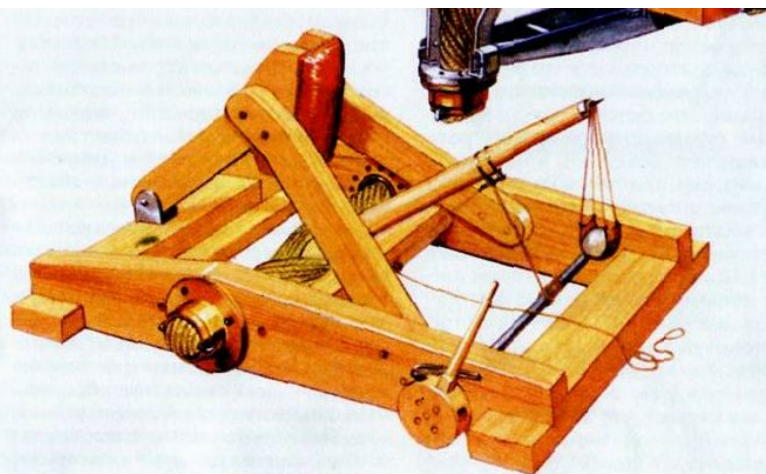
6 — трехзвездчатый наконечник стрелы от катапульты из Олинфа. Это один из нескольких наконечников, на которых выбито имя Фимитпа. Фимитп II осаждал этот город в 348 г. до н.э. Британский музей. 7 — реконструкция катапульты из Ампурияса. Такие небольшие катапульты обычно назывались «сколориннами». 8 — детали. Упрули жулы. Натяжение обеспечивалось вращением бронзовых втулок наверху и внизу.
