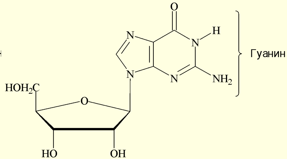
Гуанозин (G)
