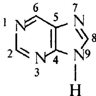
пурин
