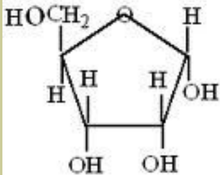
Рибоза
