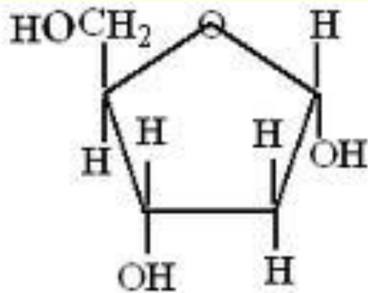
Дезоксирибоза
