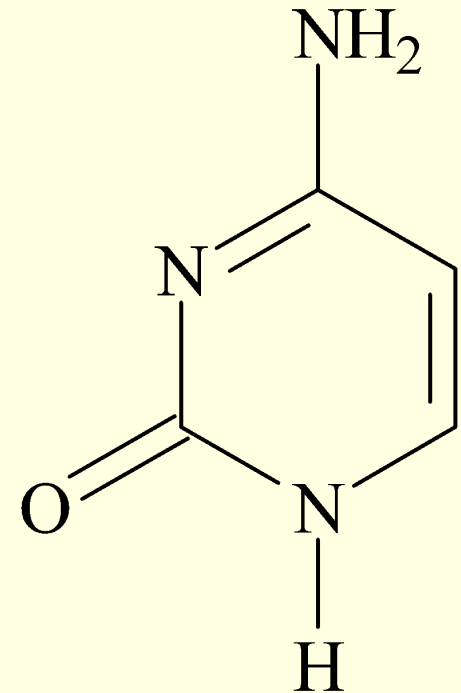
Цитозин Cyt
