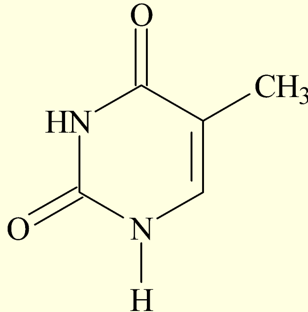
Тимин Thy
