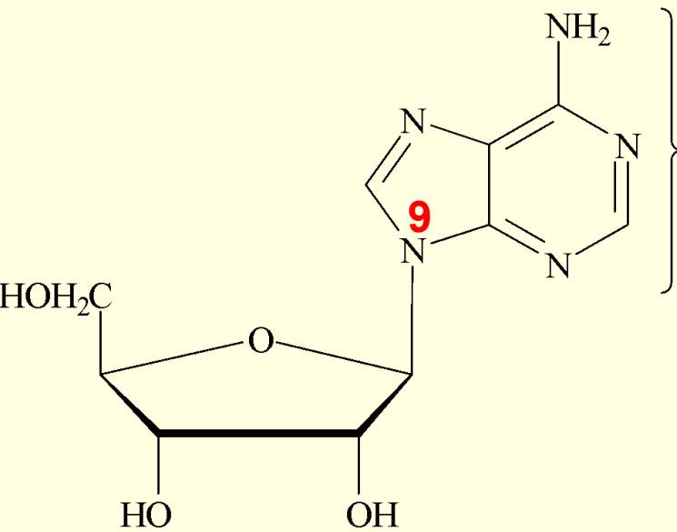
Аденозин (A)
