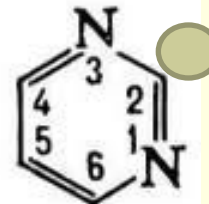
Пиримидин
