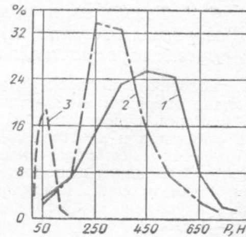
Рис. 8.36 Вариационные кривые усилий, необходимых для извлечения из почвы неподкопанных (1) и подкопанных (3) корней сахарной свеклы, и усилий (2), при которых происходит отрыв пучка ботвы от корня
