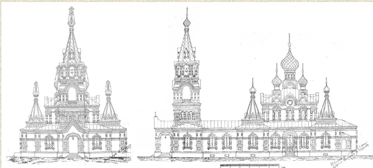
1. Чертеж храма Иоанна Богослова , нач. XX в
