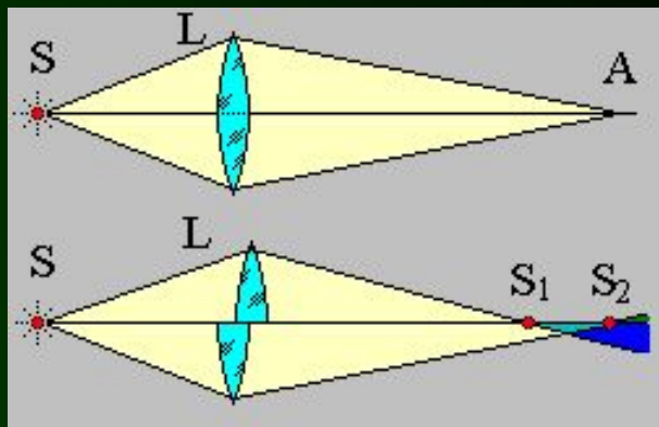
Опыт Меслина
