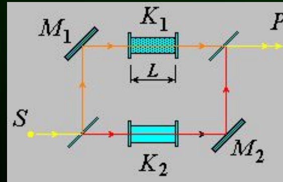
Маха – Цендера
