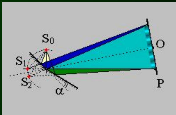
Бизеркала Френеля
