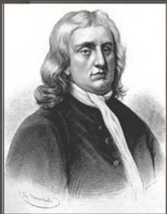
Исаак НЬЮТОН
