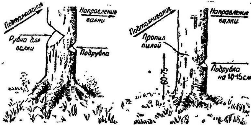
Рис. 86. Валка деревьев
