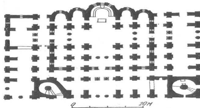
Софийский собор. План. Реконструкция Асеева Ю.С., Кресального Н.И., Волкова В.П.
