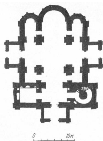
Церковь Спаса на Берестове.
