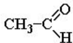
этаналь (ацетальдегид)
