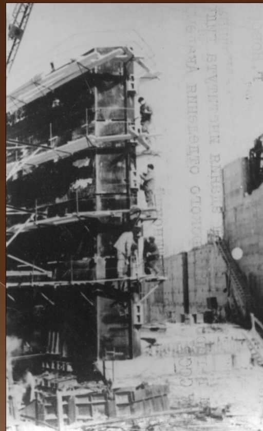
Общий вид сборки металлических двустворчатых ворот во второй камере судоходного шлюза ГЭС
