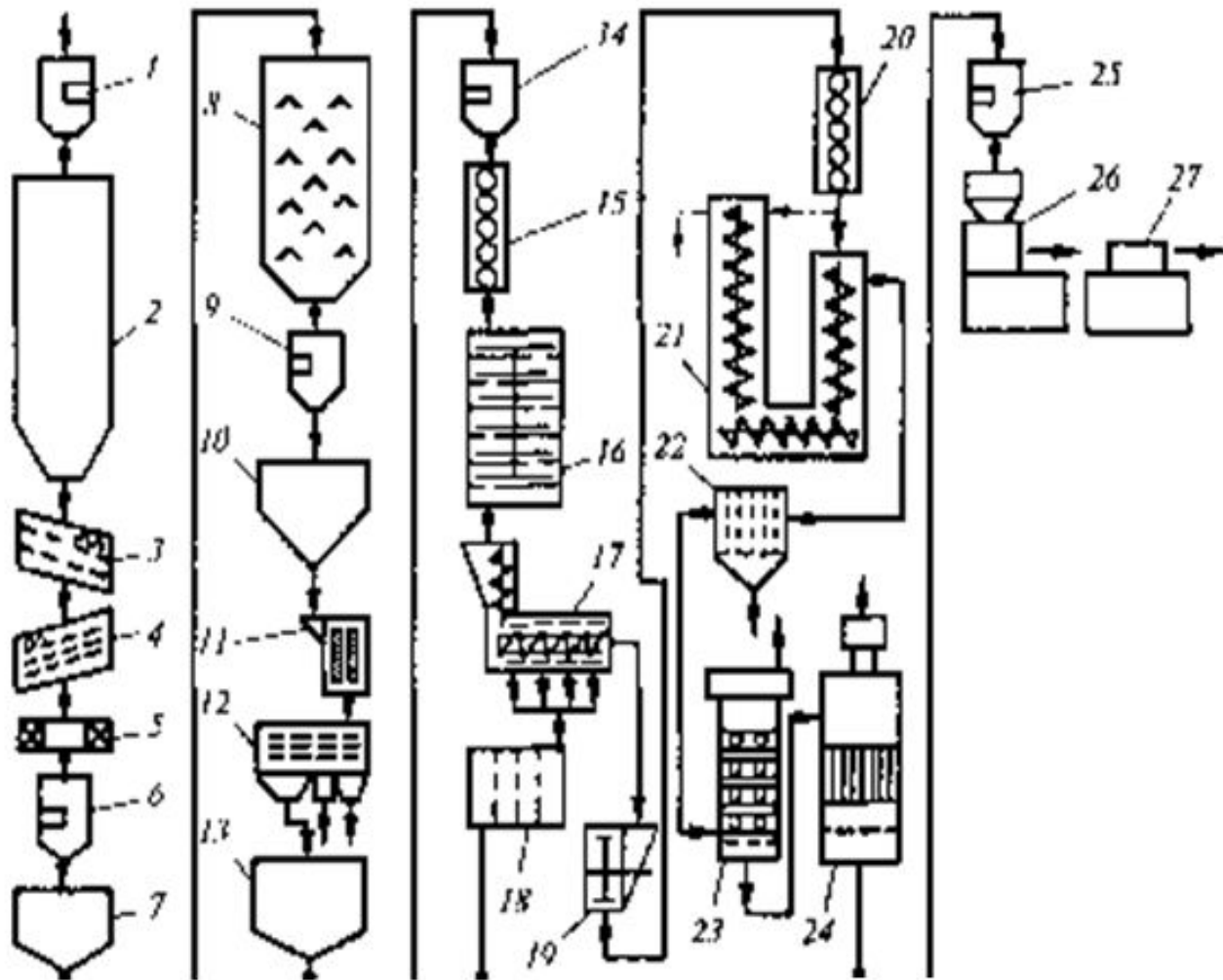
Машинно-аппаратурная схема линии производства подсолнечного масла
