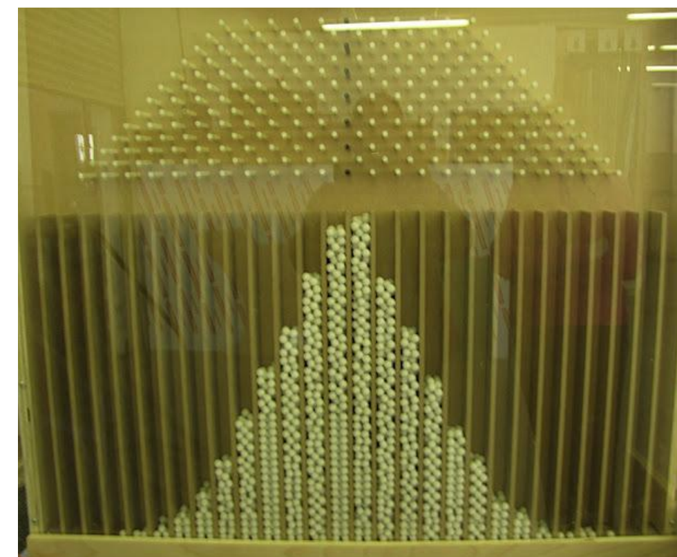
Доска Гальтона
