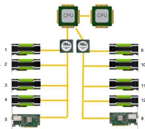
SYS-4028GR-TR(T)2
