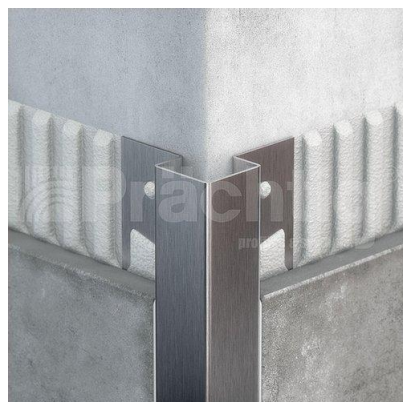
Prachting DK10/20 EM270, шлифованный, цвет серый
