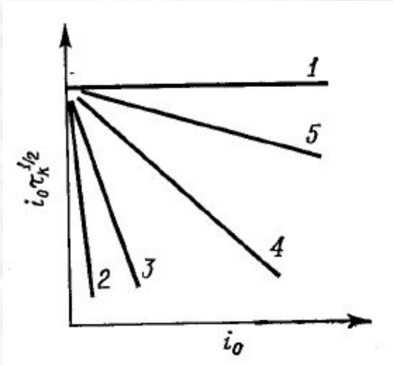
Схематическая зависимость i_0\tau_k^{1/2} от i_0 . 1 — диффузионный процесс; 2 — 5 — зависимости для увеличивающихся значений K(k_1+k_2)^{1/2} в случае электродного процесса с предшествующей химической реакцией первого порядка.
