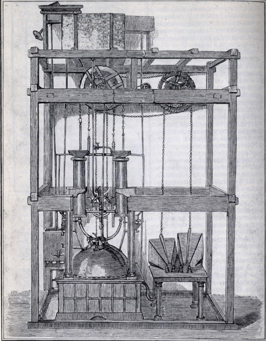
Паровая машина И. Ползунова (1763)
