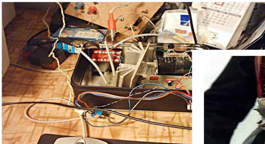
Взрывное устройство
