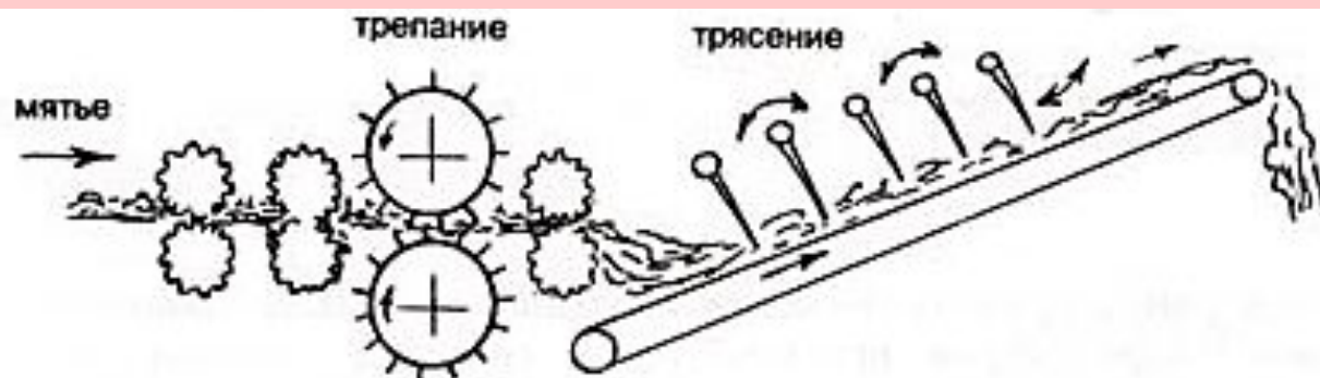
Трелание слоя сырца рифлеными вальцами
