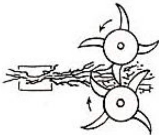
Очесывание головок
