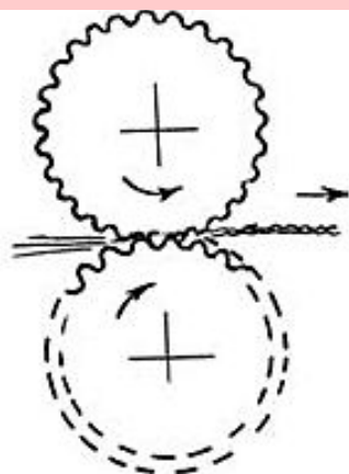
Мяте тресты
