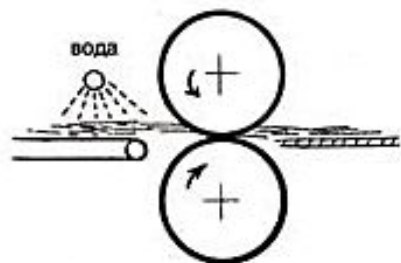
Отжим и промывка тресты
