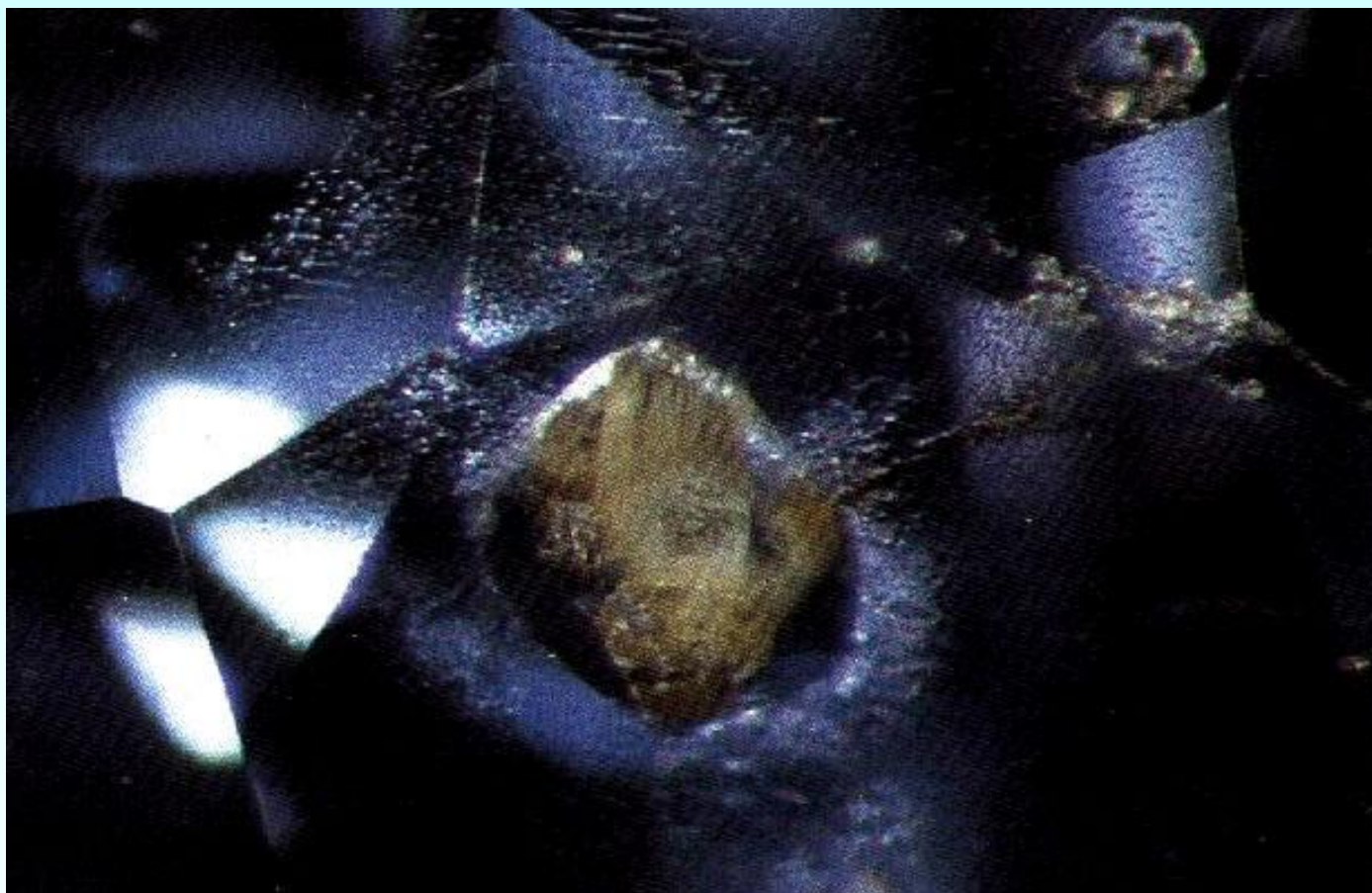
Кубический кристалл анальцима в сапфире. (Його Галч, США). Ширина картинки 0,5 мм. ( Gübelin, Koivula, 1996 )
