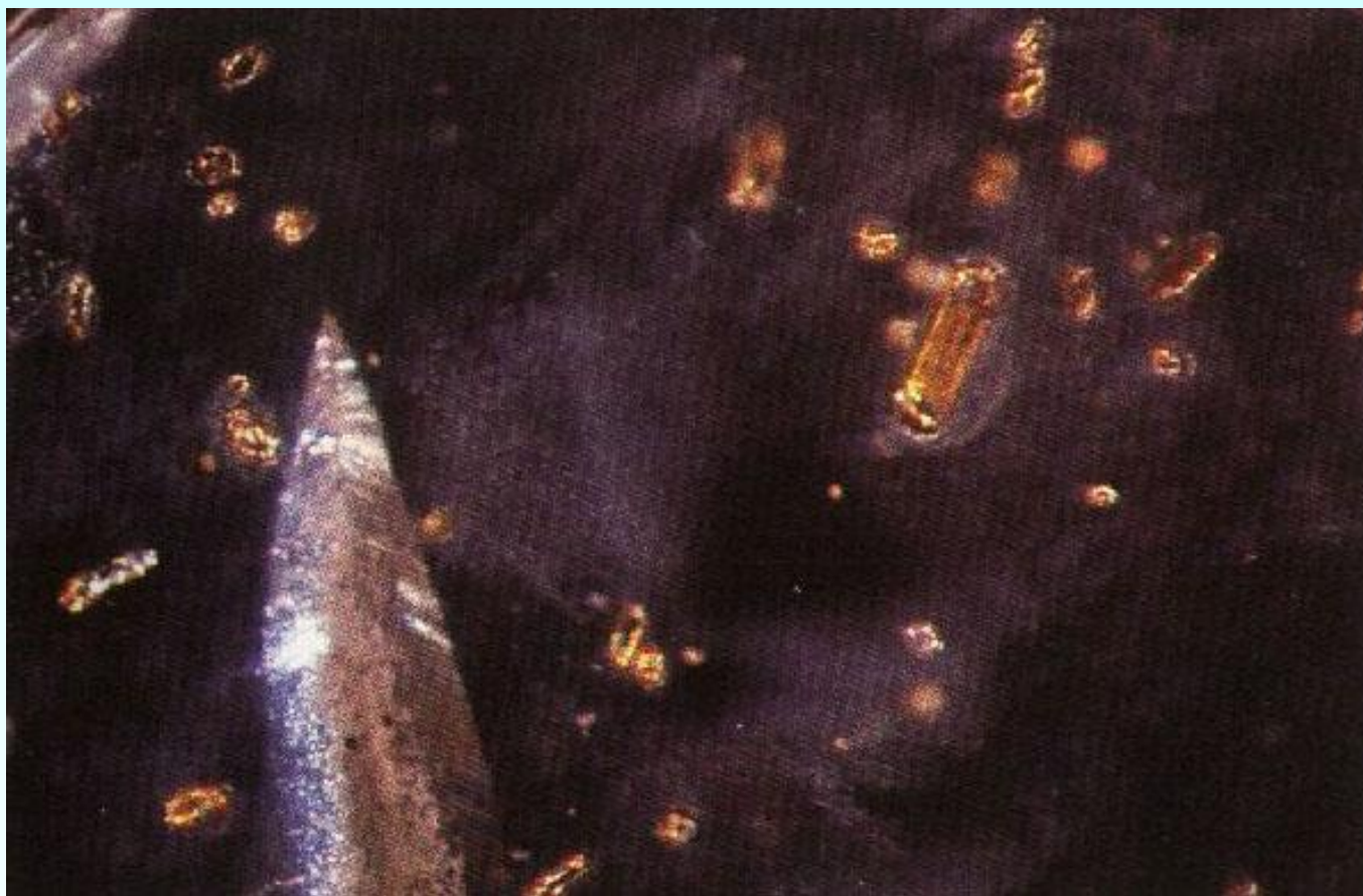
Включение кристалла доломита в сапфире (Мьянма). Ширина картинки 0,5 мм. ( Gübelin, Koivula, 1996 )
