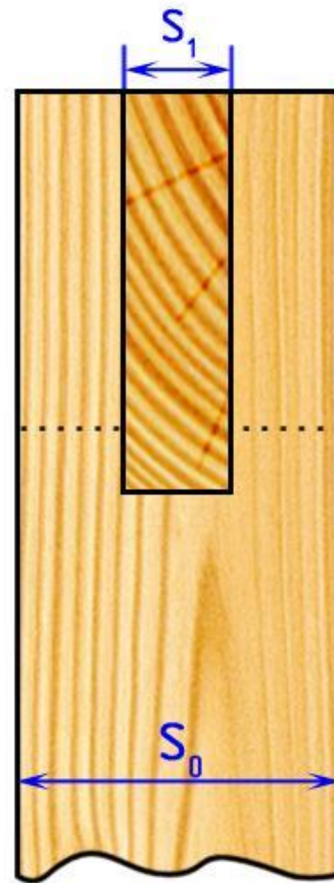
Угловое концевое на ус со вставным сквозным плоским шипом УК-11
