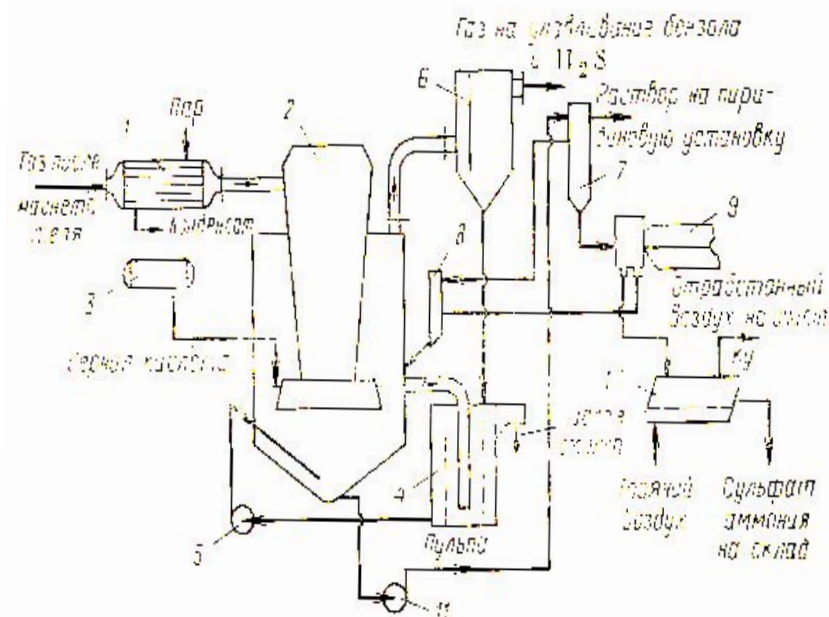
Технологическая схема получения сульфата аммония:
