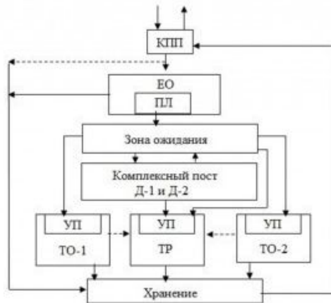
Схема технологического процесса ТО и ТР
