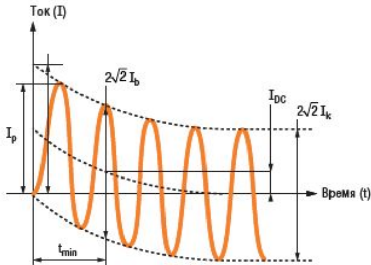
Рис. С5: Графическое представление величин короткого замыкания согласно МЭК 60909
