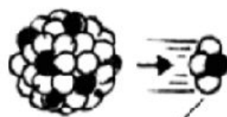
Альфа-частица
