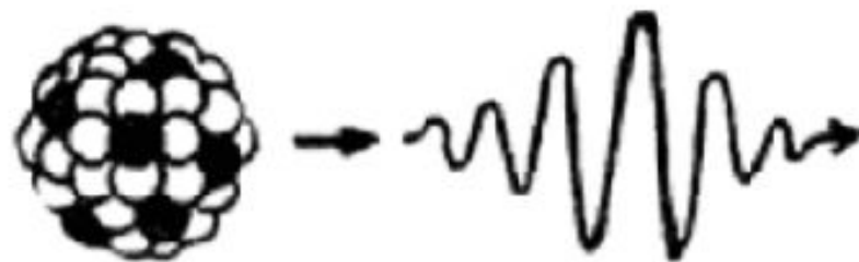
Гамма-квант
