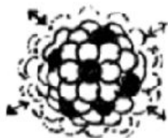
Возбуждённое ядро
