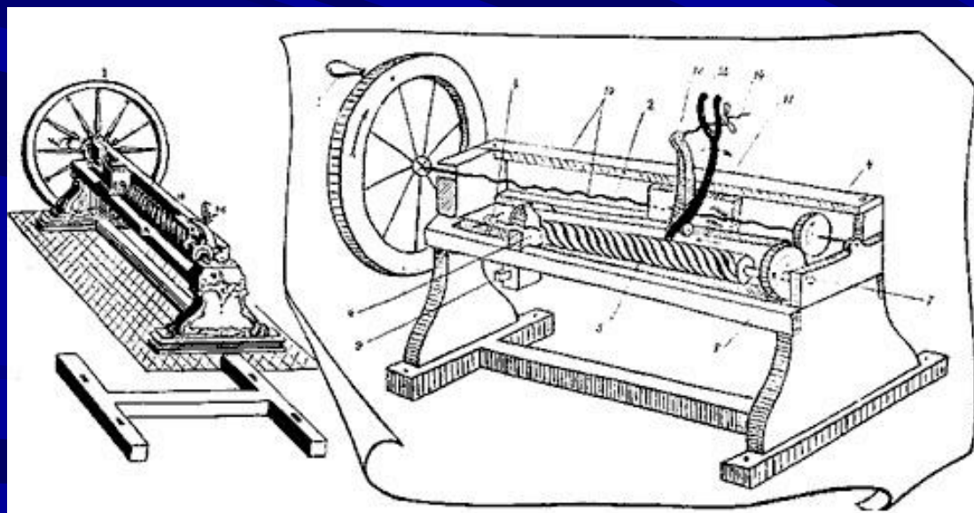
Винторезный станок А.К. Нартова
