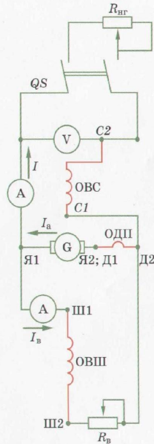
Генератор смешанного возбуждения
