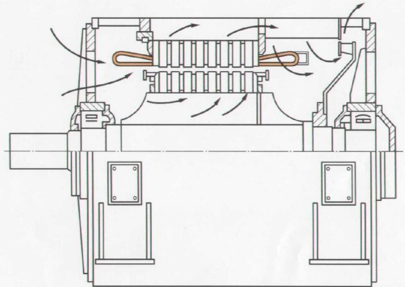
Схема вентиляции асинхронного двигателя АН2
