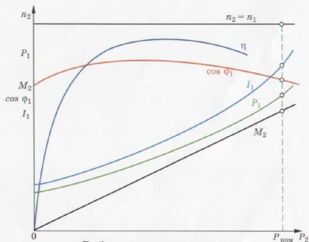
Рабочие характеристики синхронного двигателя
