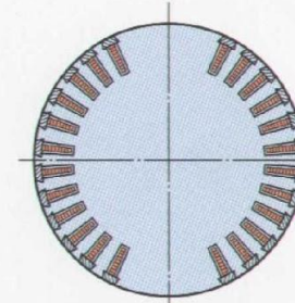
Неявнополюсный ротор
