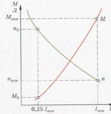
Рабочие характеристики двигателя последовательного возбуждения
