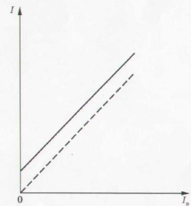
Характеристика короткого замыкания
