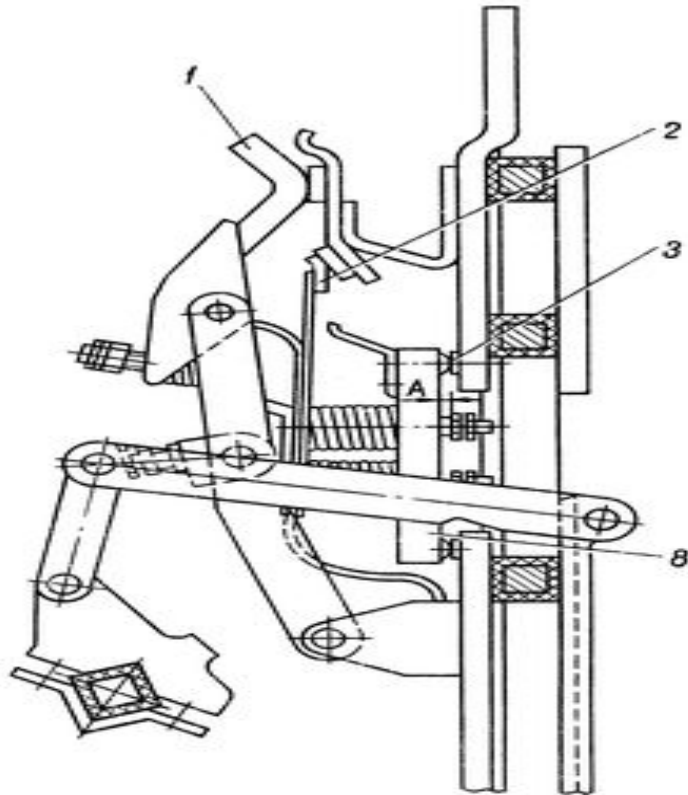
Рисунок 1. Контактная система во включенном положении;
