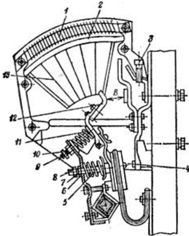
Рисунок 1. Контактная система и дугогасительная камера автоматических выключателей АВМ-15
