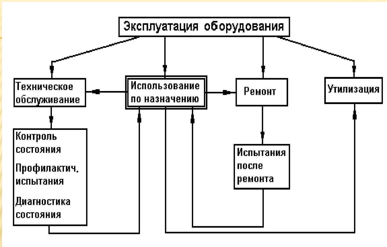
Рисунок 1-Схема технической эксплуатации электрооборудования
