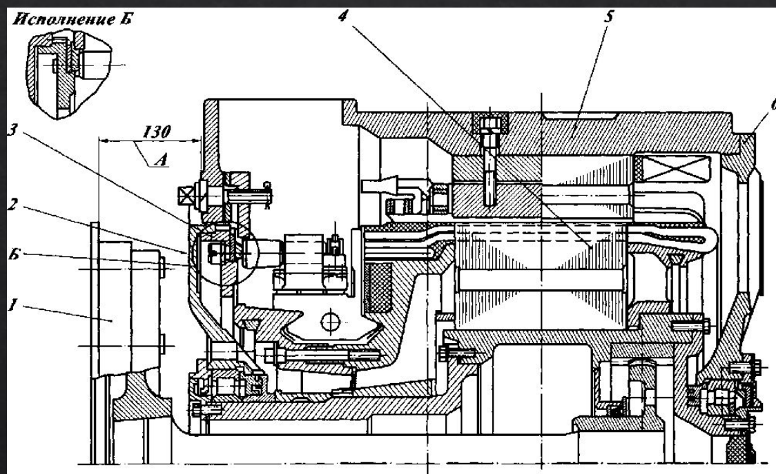
Продольный разрез тягового двигателя НБ-520В
