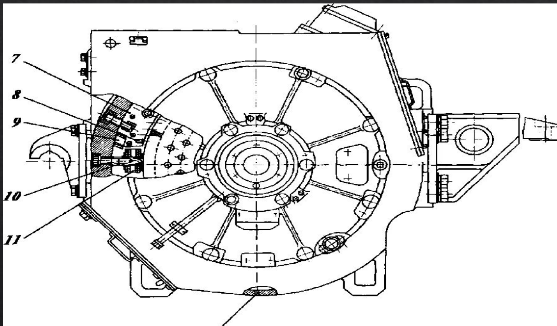
Поперечный разрез тягового двигателя НБ-520В
