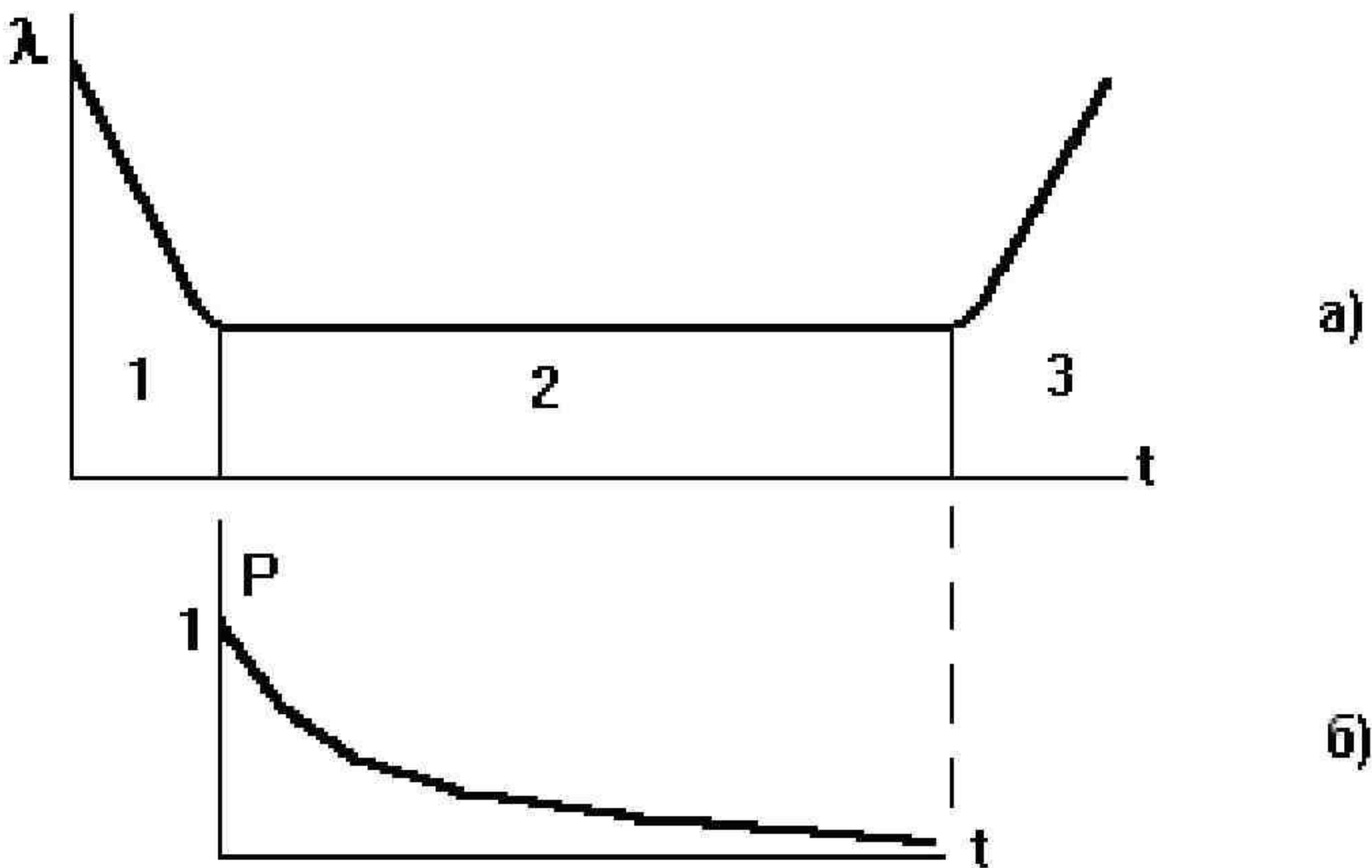
Рисунок 3-График зависимости интенсивности отказов от времени эксплуатации (а) и распределение вероятности безотказной работы оборудования (б)
